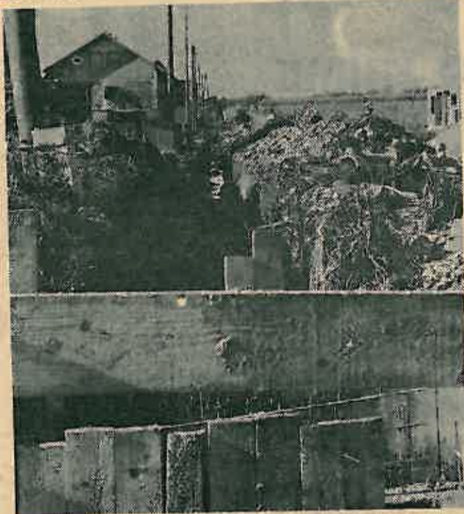
Radovi se izvode planski, najprije se kopaju rovokopačima kanali da bi se nakon tog odmah drugi dan prišlo montiranju i polaganju cijevi.
