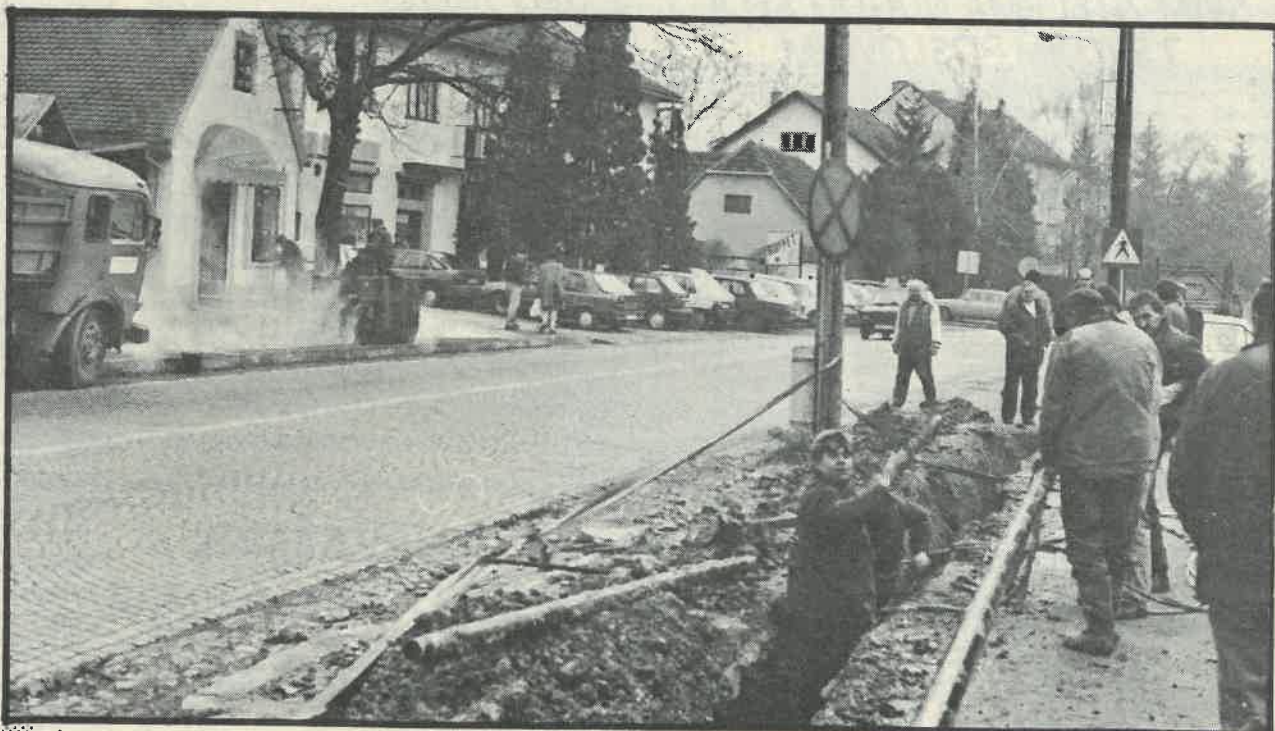
Istovremeno radovi s obje strane kolnika
